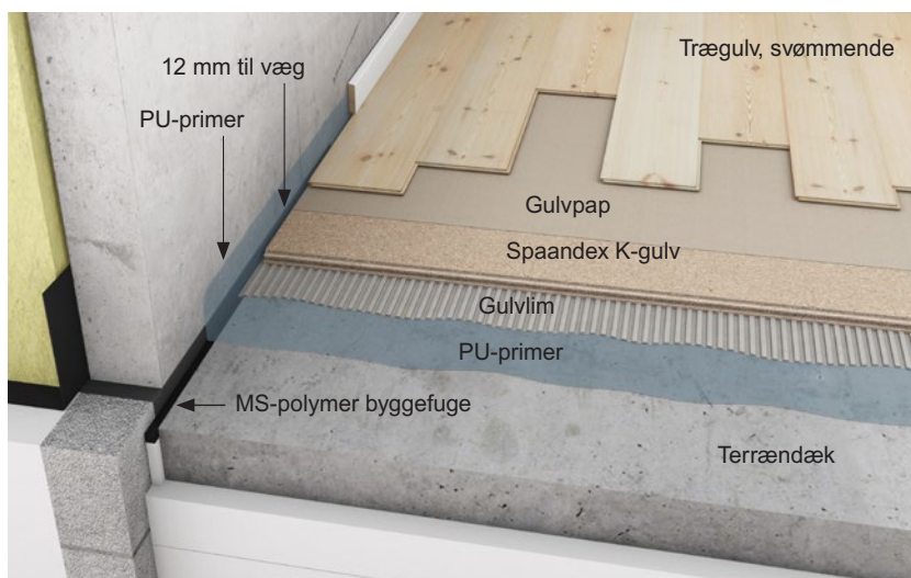
Figur 2 Spaandex K-gulv fuldlimet til terrændæk og udført med svømmende trægulv. Fugtbeskyttet af 2-3 lag PU-primer og radonspærre af MS-polymer byggefuge mellem væg og terrændæk
