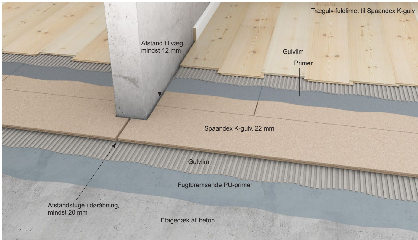
Figur 1 Spaandex K-gulv fuldlimet til etagedæk af beton og udført med fuldlimet trægulv.
